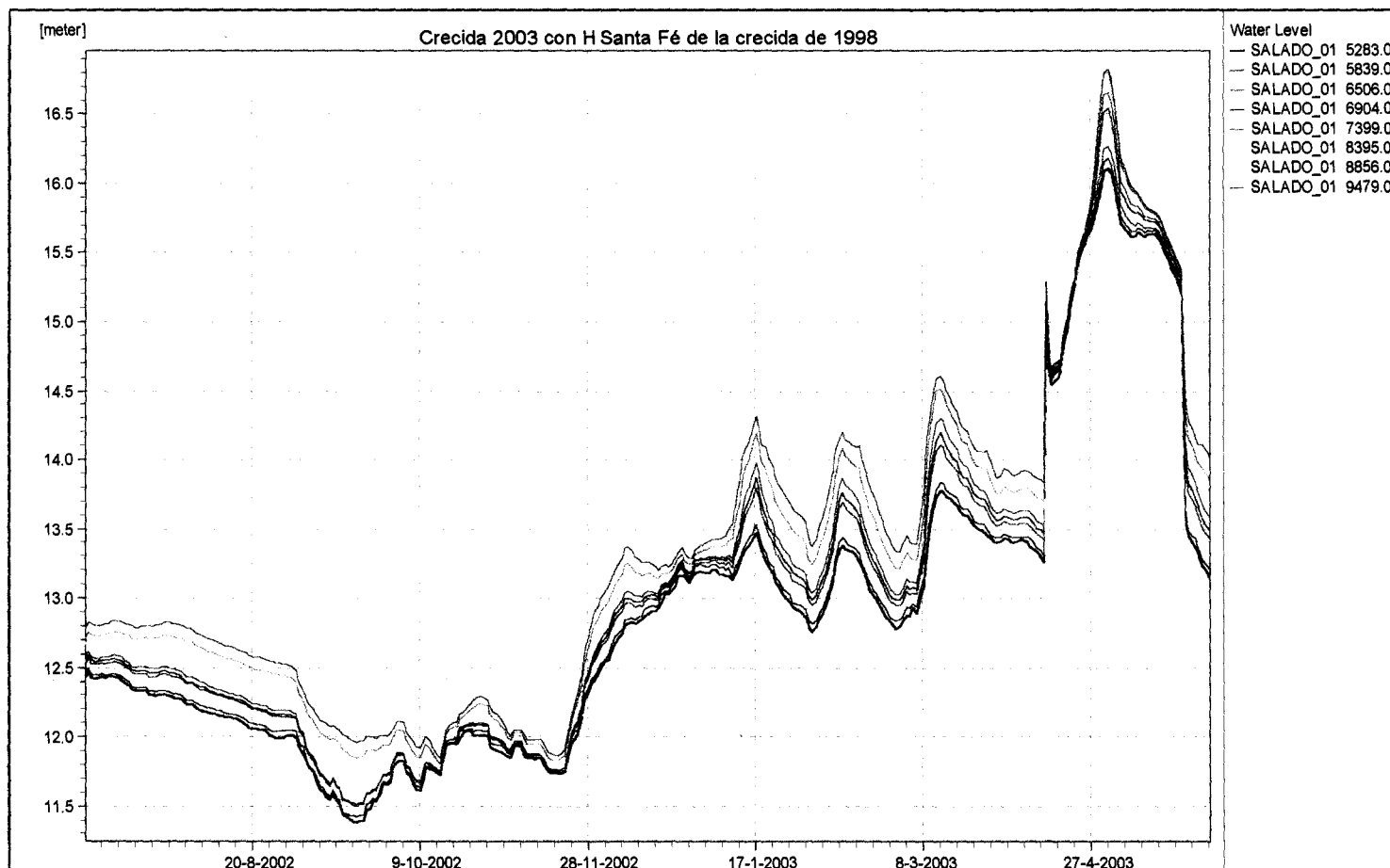
Figura 7.27 Cálculo de alturas modelo HD crecida 2003 con H Santa Fé año 1998.
