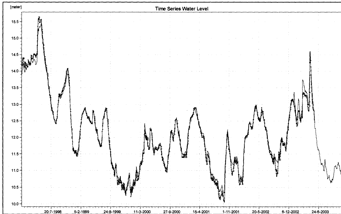
Figura 7.21 Verificación del modelo HD , alturas de agua en escala Inali Valores calculados en rojo , Valores medidos línea azul.
