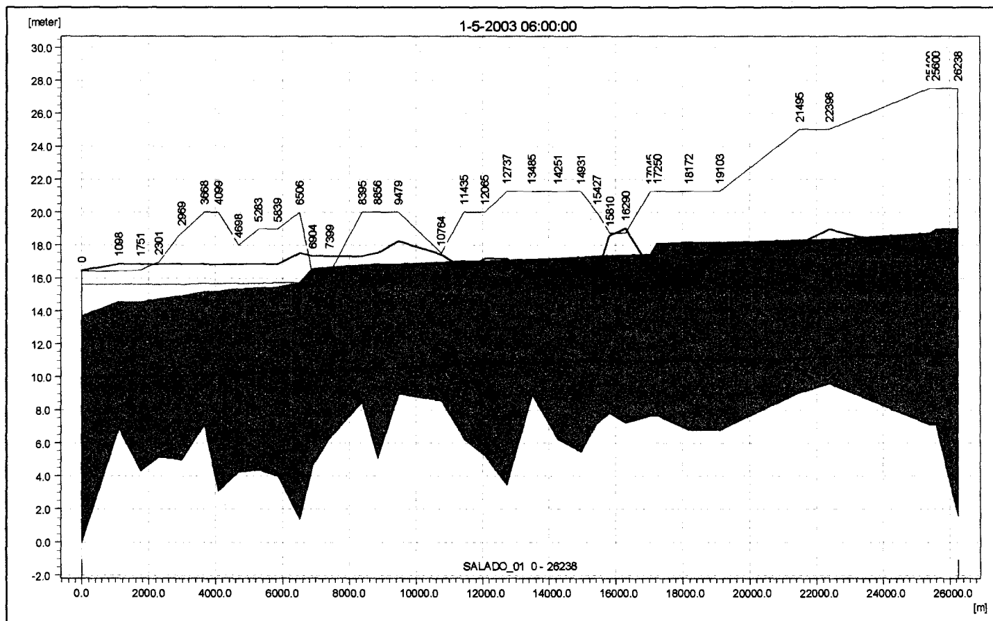
Figura 7.22 Verificación del modelo HD , Perfil de alturas fecha 1 de mayo 2003 desde Coronda a RP 70.
