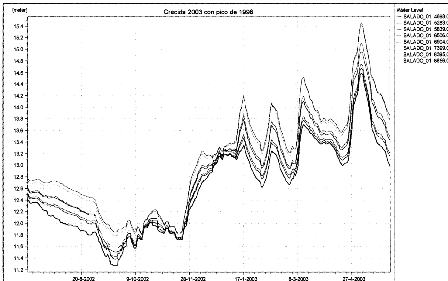
Figura 7.26 Cálculo de alturas modelo HD crecida 2003 con Q RP 70 año 1998.
