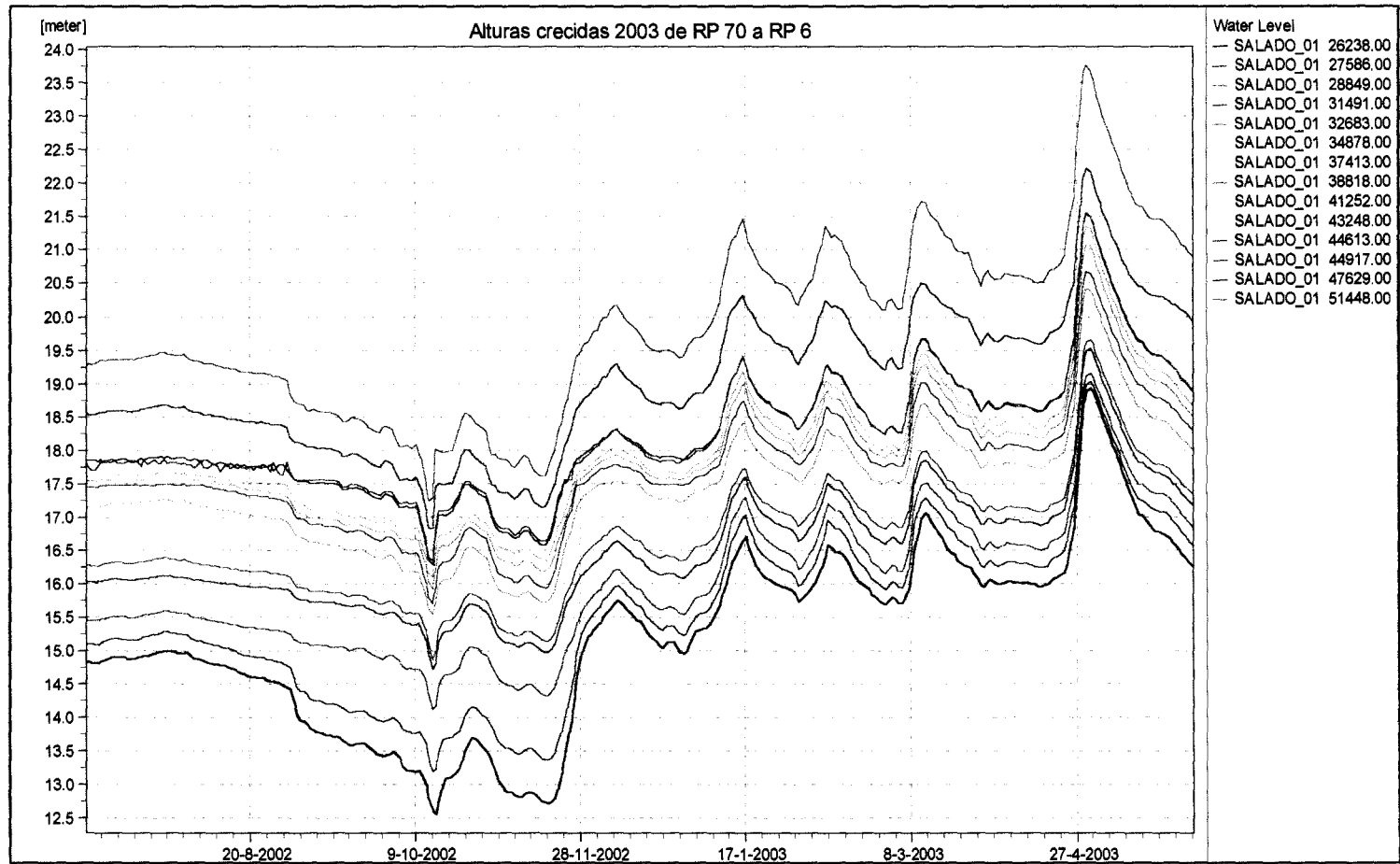
Figura 7.25 Cálculo de alturas modelo HD crecida 2003 desde RP 70 a RP 6.
