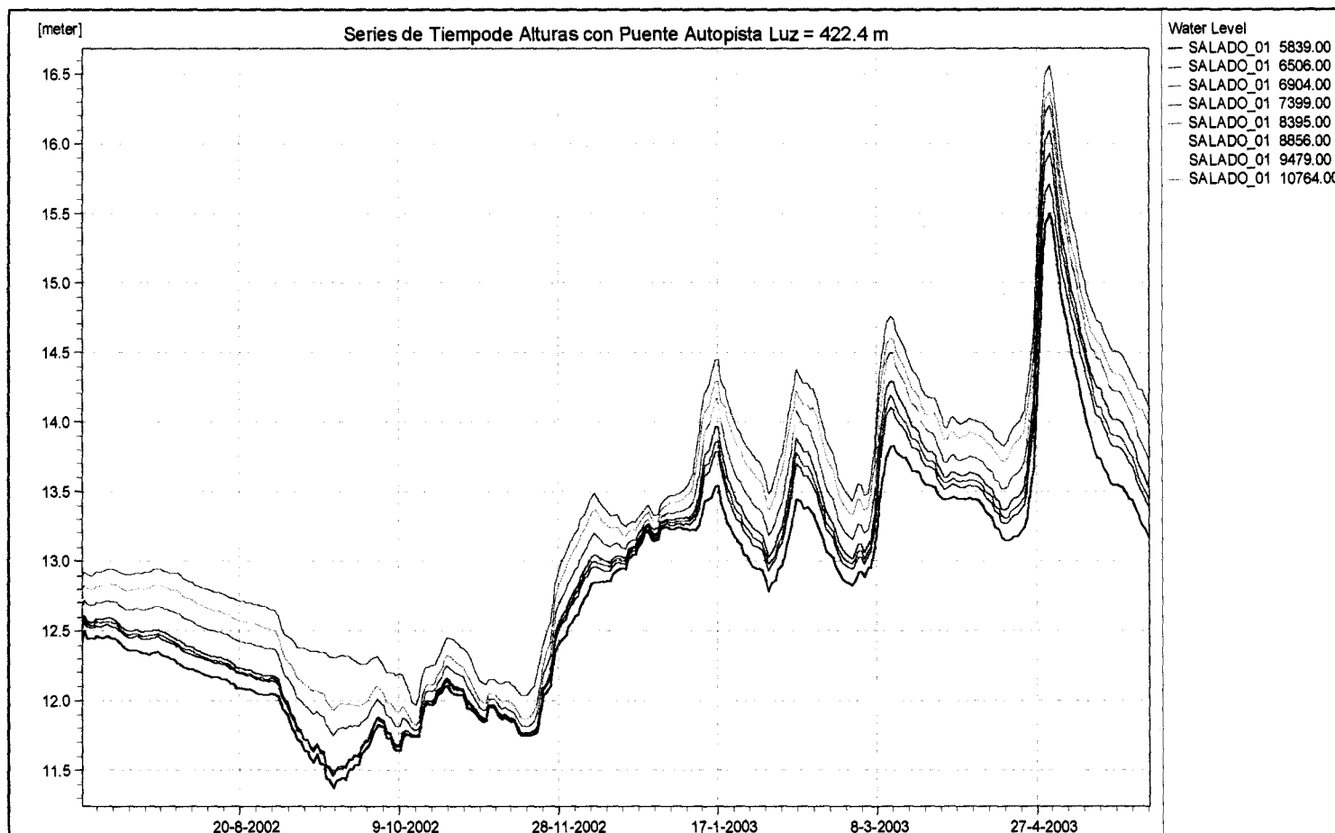
Figura 7.24 Cálculo de alturas modelo HD con puente Autopista L = 422.4 metros
