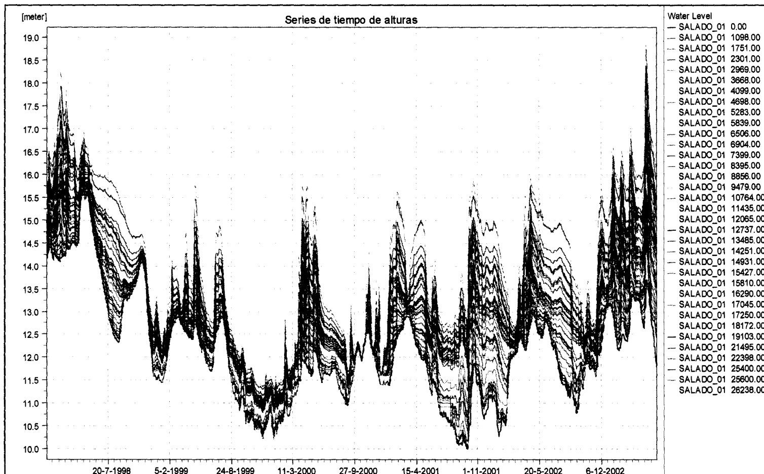
Figura 7.23 Cálculo de alturas modelo HD , período enero 1998 a junio 2003.
